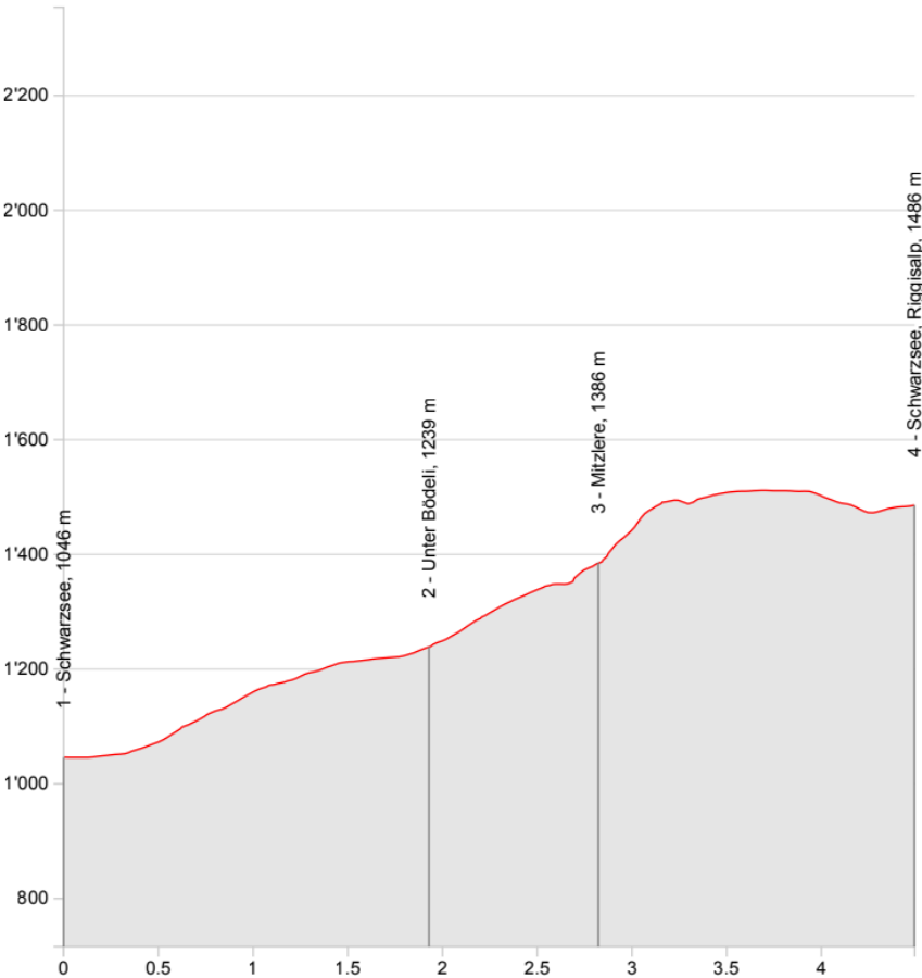
Profil d'élévation
